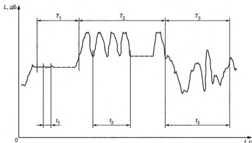
L — уровень шума как функция времени; T_1 — продолжительность рабочей операции 1; T_2 — продолжительность рабочей операции 2; T_3 — продолжительность рабочей операции 3; t_1 — длительность измерения шума операции 1 (почти постоянный шум); t_2 — длительность измерения шума операции 2 (почти периодический шум); t_3 — длительность измерения шума операции 3 (непостоянный шум)
